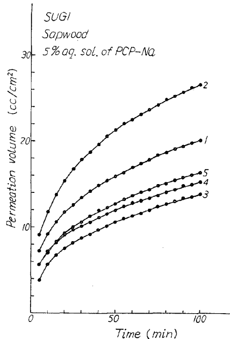
Fig. 2-4. Permeation courses.
