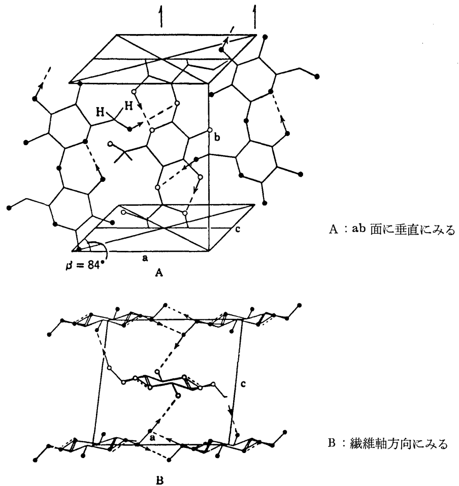
図-6 セルロース I 単位胞中の分子内、分子間水素結合を示す図 (Liang, Marchessault による) 26)
