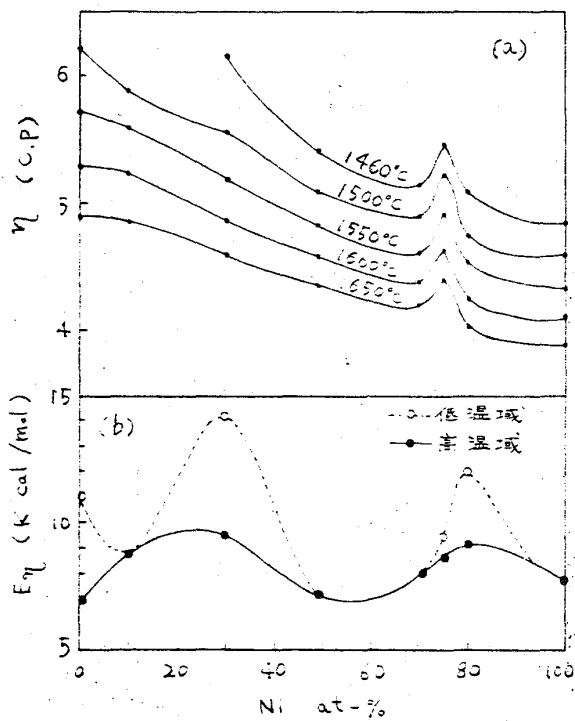
Fig. 5 Fe-Ni 合金の粘度 (a) と粘性流動の活性化エネルギー (b)
