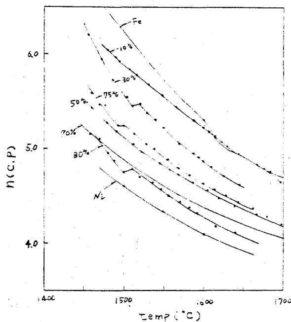
Fig. 1 Fe-Ni 合金の粘度
