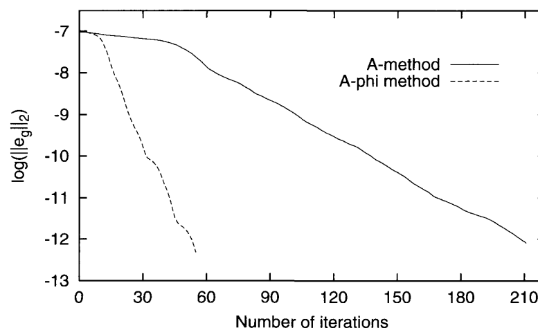
図2 導電性領域における curl の Null 空間に属する誤差の振る舞いの比較
