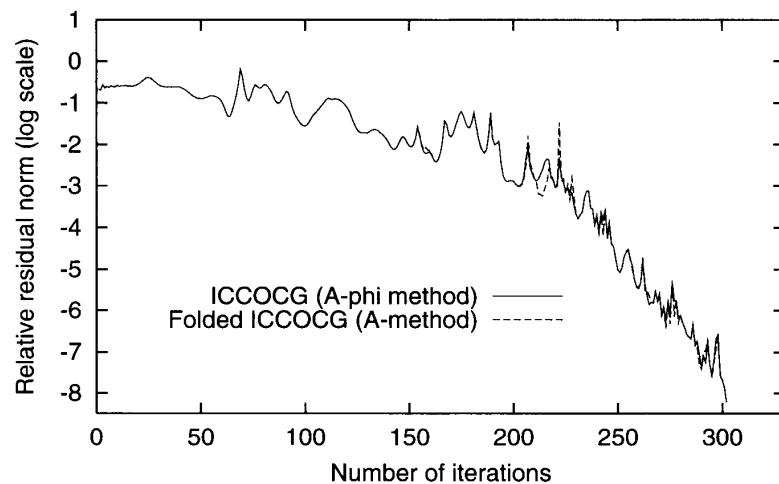
図3 A- \phi 法における ICCOCG 法と A-法における Folded ICCOCG 法の残差収束における等価性
