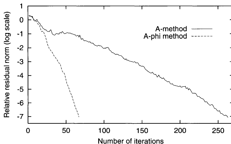
図1 A-法と A- \phi 法における残差の収束過程の比較
