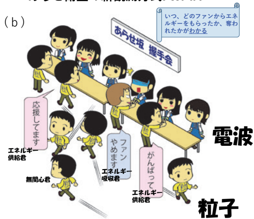
図3: 電波と粒子のエネルギーのやりとりを観測する手法の比較 (イラスト: のし)
