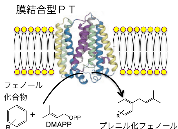
図2: 植物プレニル基転移酵素 (PT) によるフェノールの修飾反応
