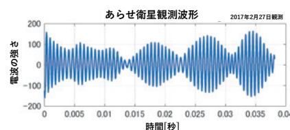
図2: あらせ衛星に搭載されたプラズマ波動観測器(PWE)で観測された放射線帯で発生している電波の波形
