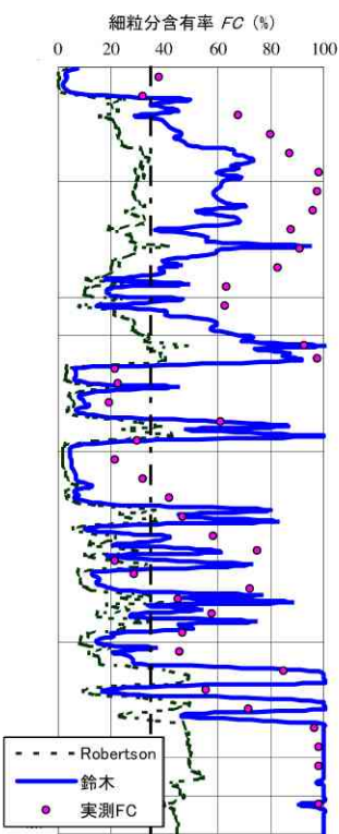
図-7 細粒分含有率 FC の推定
