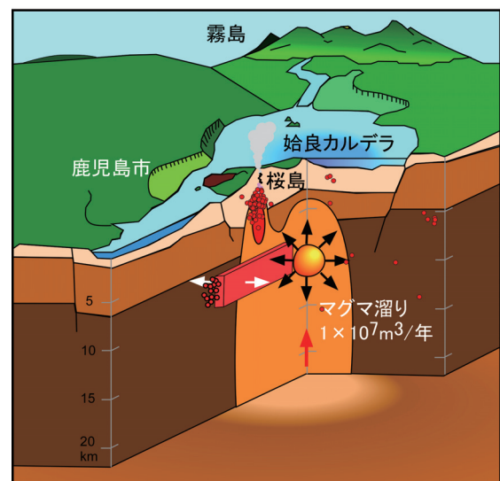
地球物理学的観測から推定される 桜島のマグマ供給系
