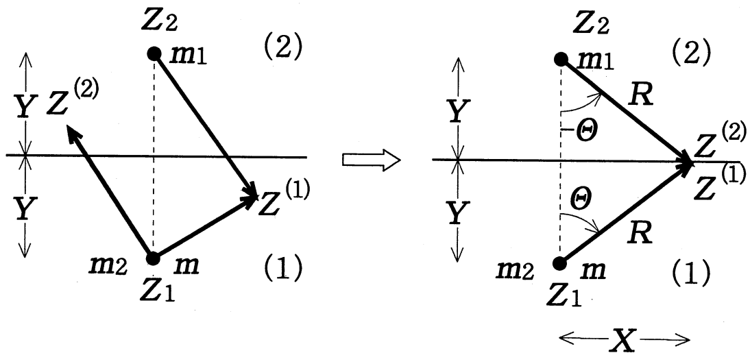
図 1: 磁気単極子による磁気ポテンシャル決定のための鏡像法．領域 (1) では m(Z_1) と m_1(Z_2) より，領域 (2) では m_2(Z_1) より磁気ポテンシャルを構成し（左図），境界面上の点 Z^{(1)} = Z^{(2)} = Z_1 + X + iY = Z_2 + X - iY で連続条件 (5) を満たすように m_1, m_2 を定める（右図）．
