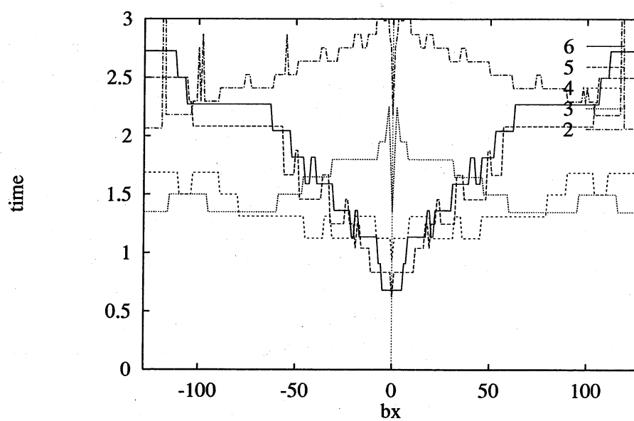
図 5. MGCGS 法で計算したときの解が収束するまでの計算時間
