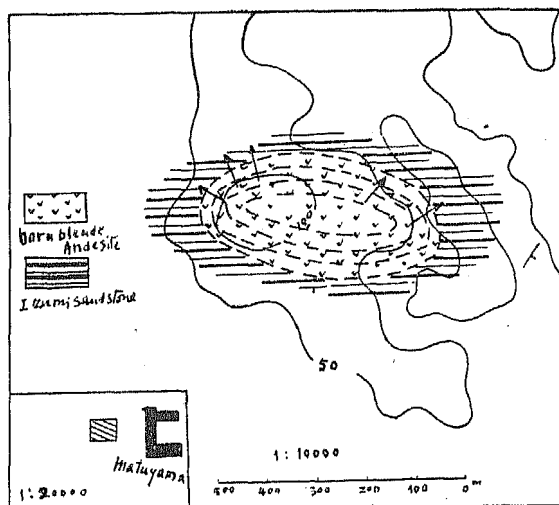
第二圖 安山子山岩の對流組織
