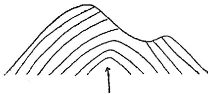
第三圖 岩石の節理構造(北側)
