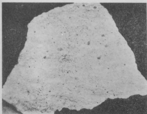
圖一第 岩子山安山岩の對流組織
