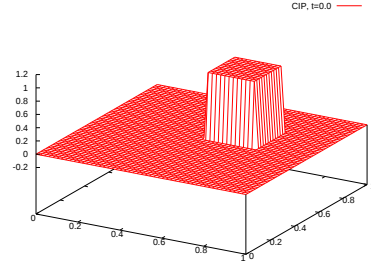
CIP t = 0
