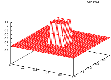
CIP t = 0.5
