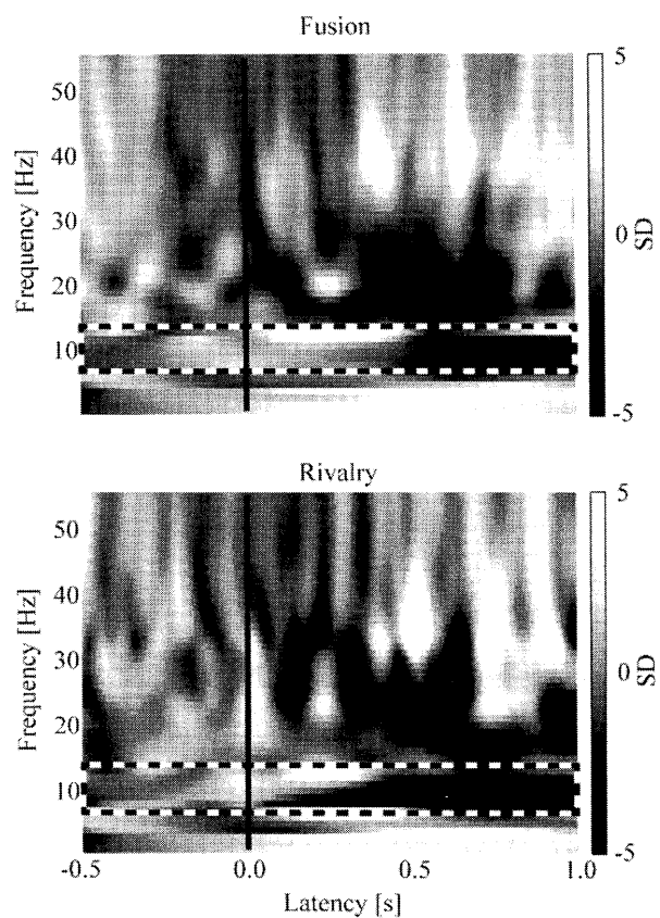
図 7. Fusion 運動と Rivalry 運動における Cz でのパワーの時間一周波数マップ. 破線内は注目する周波数帯 (8-13 Hz).
