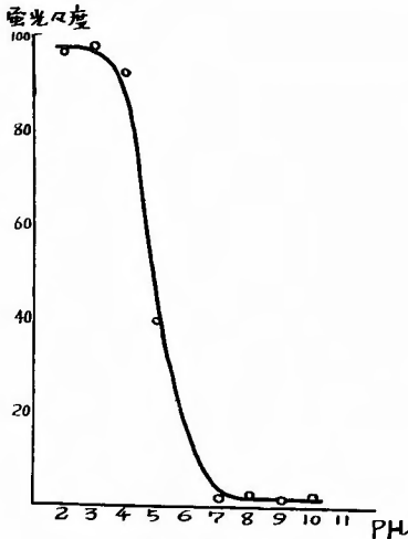
第2図 NA のアルミナへの吸着曲線。300γ/dl NA-水溶液 100cc に EDTA 1g, Alumina 2.5g 5) を加え、pH を 0.5N-NaOH で調整しながら、各 pH でその上清をとり螢光々度をみる。Aでも同様の曲線である。
