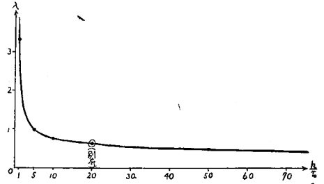
第4圖 埋設深度と \lambda (相對値)
