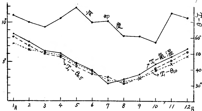
第7圖 研究所引湯冷却度の年變化と氣溫又は地溫の影響
