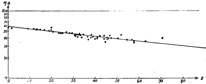
第5圖 別府引湯の T-\theta と s との関係
