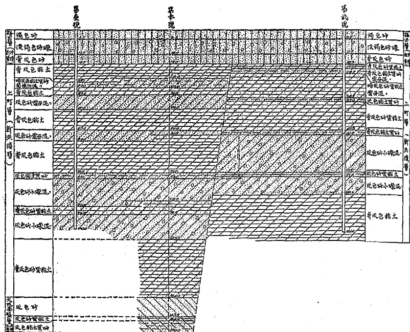
南區日本橋筋三丁目某大商店敷地斷面圖
