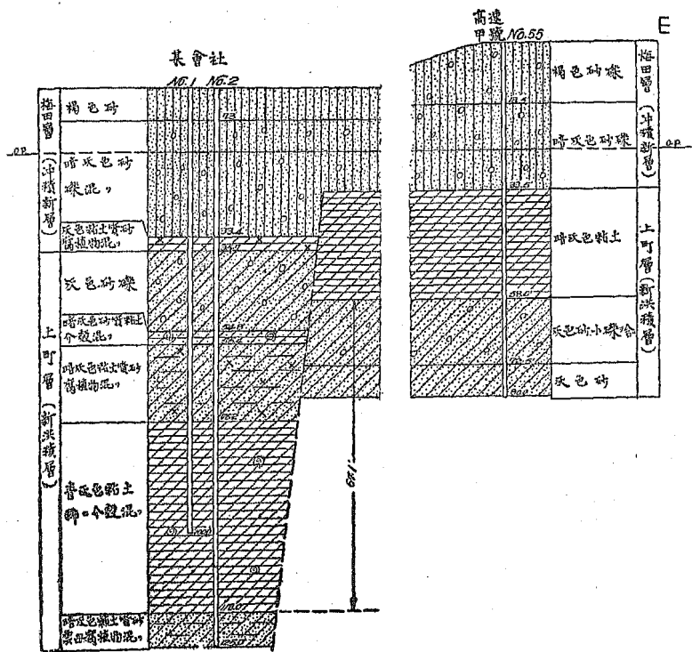
東區界筋備後町某會社敷地斷面圖
