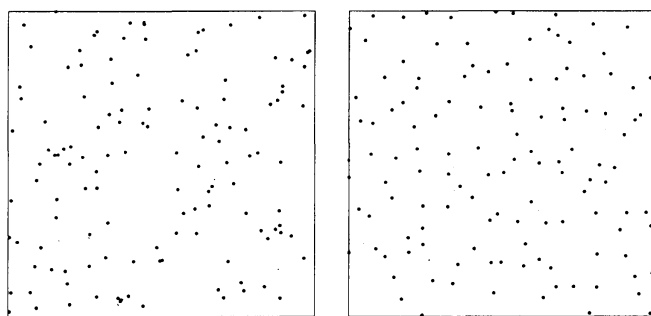
図 1 左: ポアソン点過程, 右: 行列式点過程 (Ginibre 行列の固有値)
