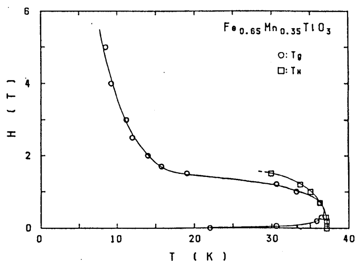
x=0.65の試料における T_0 、 T_N の磁場依存性
