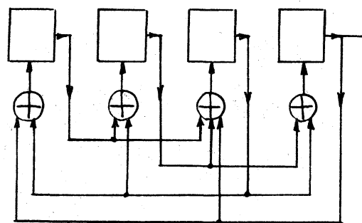
図2. F^5 に対応するシフトレジスタ
