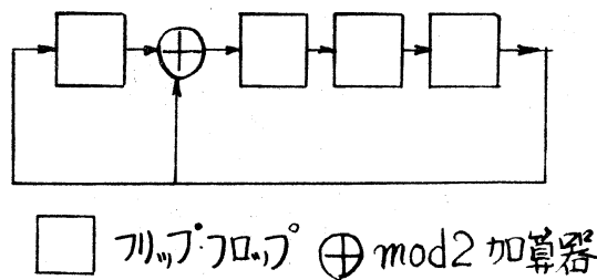
図1. 式(8)のF行列に対応する フィードバック・シフトレジスタ
