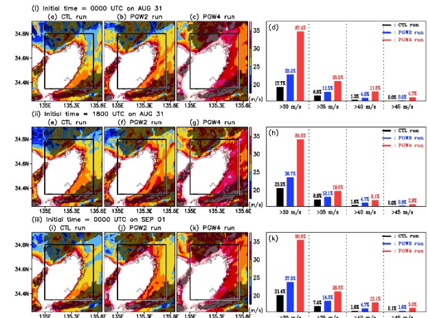
図 8. (a-c) 初期時刻が 2018 年 8 月 31 日 00 UTC の (a) CTL run、(b) PGW2 run、(c) PGW4 run から得られた期間最大風速の空間分布図。ただし、陸上のみを描画している。灰色の陰影は、標高が 100 m を超える地域を表す。(d) 大阪湾周辺（図 8a-c の黒枠内）の標高 100 m 未満の平野部で領域平均した期間最大風速がある閾値（30、35、40、45 m/s）を超える領域が、注目している平野部全体に占める割合。黒、青、赤色の棒グラフは、それぞれ CTL run、PGW2 run、PGW4 run の結果を表す。(e-h) 図 8a-d と同様であるが、初期時刻が 2018 年 8 月 31 日 18 UTC の結果。(i-k) 図 8a-d と同様であるが、初期時刻が 2018 年 9 月 1 日 00 UTC の結果。
