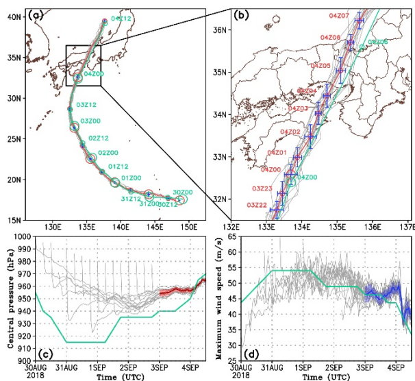
図 2. (a) WRF (灰線: 各アンサンブルメンバー、赤線: アンサンブル平均) と気象庁ベストトラックデータ (緑線) から得られた TC1821 の経路。各日 00 と 12 UTC の TC1821 の位置を丸印で示している。青十字は、メンバー間の経路のばらつき ( \pm 1\sigma ) を表す。(b) 図 2a と同様であるが、図 2a の黒枠内を拡大した図。(c) WRF (灰線: 各アンサンブルメンバー、赤線: アンサンブル平均) と気象庁ベストトラックデータ (緑線) から得られた TC1821 の中心気圧の時系列図。陰影は、メンバー間の中心気圧のばらつきを表す。(d) 図 2c と同様であるが、最大風速の時系列図。
