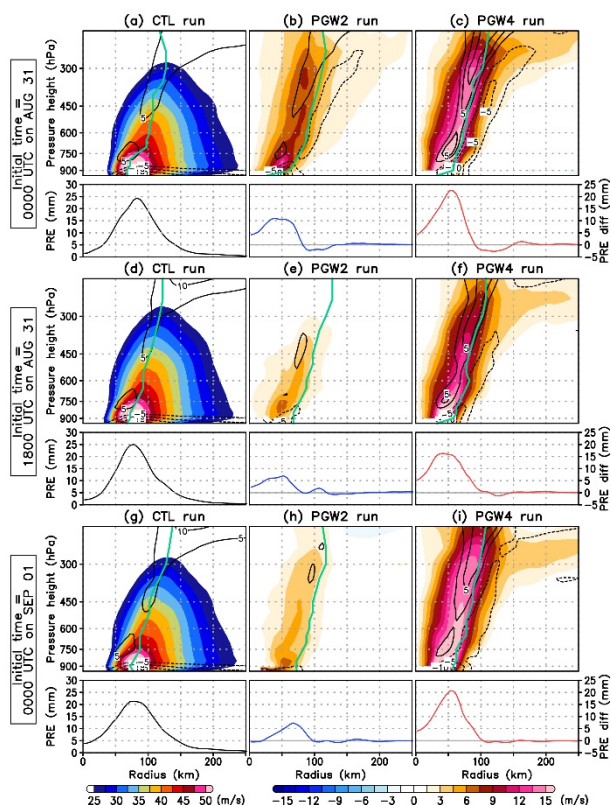
図6. (a-c) 初期時刻が 2018 年 8 月 31 日 00 UTC における (a) CTL run、(b) PGW2 run、(c) PGW4 run から得られた上陸直前の方位角した接線風速(陰影)と動径風速(等値線)の半径高度断面図。緑線は各高度の RMW を表す。下段のグラフは、1 時間降水量の動径分布を示す。PGW run は、RMW を除いて CTL run との差 (PGW minus CTL) として描画。(d-f) 図 6a-c と同様であるが、初期時刻が 2018 年 8 月 31 日 18 UTC の結果。(g-i) 図 6a-c と同様であるが、初期時刻が 2018 年 9 月 1 日 00 UTC の結果。
