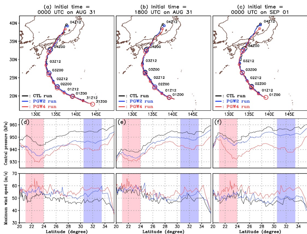
図5. (a-c) 初期時刻が (a) 2018 年 8 月 31 日 00 UTC、(b) 2018 年 8 月 31 日 18 UTC、(c) 2018 年 9 月 1 日 00 UTC における CTL run (黒線)、PGW2 run (青線)、PGW4 run (赤線) から得られた TC1821 の経路。各日 00 と 12 UTC の台風の位置を丸印で示している。(d-f) 各初期時刻の各数値実験から得られた TC1821 の中心気圧(上段)と最大風速(下段)の時系列図。横軸は緯度を表す。赤(青)の陰影は、最盛期(上陸直前)の緯度帯を表す。
