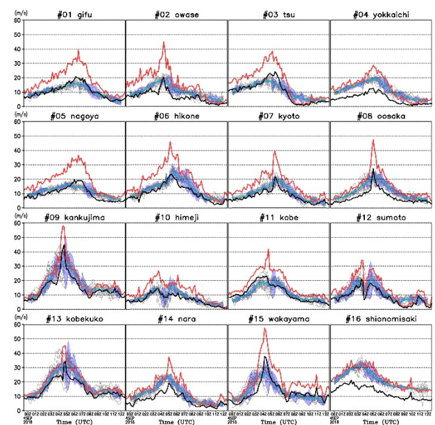
図 3. 観測された瞬間風速 (赤線) と平均風速 (黒線) の時系列図。WRF の結果 (灰線: 各アンサンブルメンバー、青線: メンバー平均) も併せて描いている。陰影は、メンバー間の地上風速のばらつきを表す。各図の数字は、図 1b の丸印に対応する。
