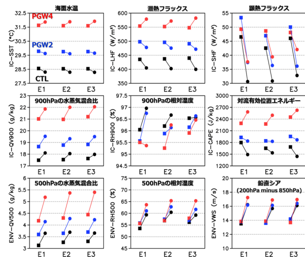
図 7. 最盛期（丸印）と上陸直前（四角印）における環境場パラメータ。黒色は CTL run、青色は PGW2 run、赤色は PGW4 run を表す。IC-（ENV-）は、台風中心から半径 200（600）km 以内で領域
