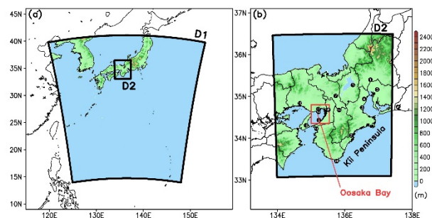
図 1. WRF における計算領域。陰影は、標高を表す。図 1b の丸印は、図 3 の各観測点の位置に対応する。
