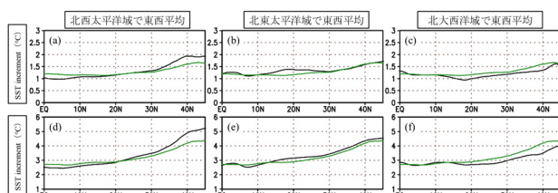
図 4. (a-c) d2PDF から得られた (a) 北西太平洋域、(b) 北東太平洋域、(c) 北大西洋域で東西平均した 9 月の SST increment（黒線）。SST increment の全球平均値も緑線で併せて描いている。(d-f) 図 4a-c と同様であるが、d4PDF における 9 月の SST increment。
