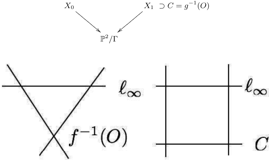
図1 X_0 と X_1
