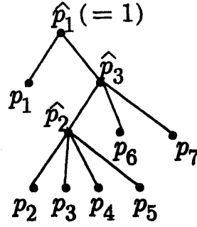
図 1: 7 個の葉と 3 個の内節点をもつ根付き木
