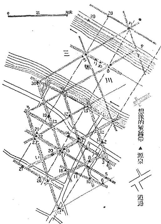
第三圖 三朝村に於ける源泉の配置を示す
