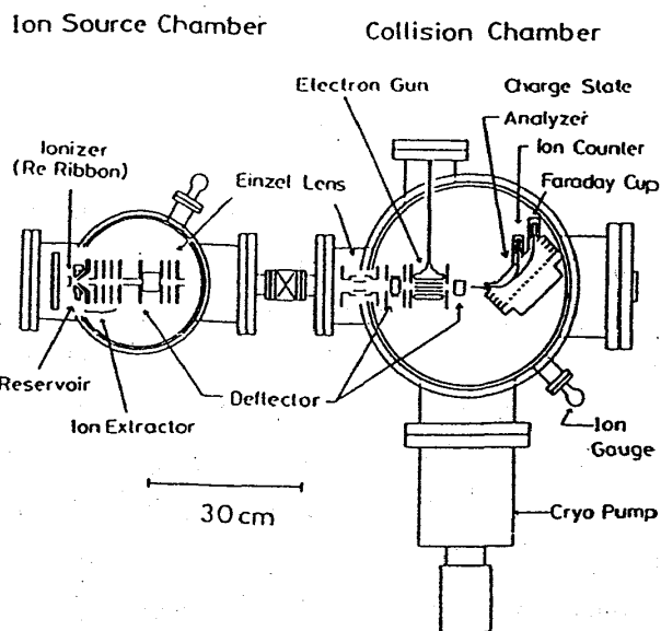
図2. 実験装置
