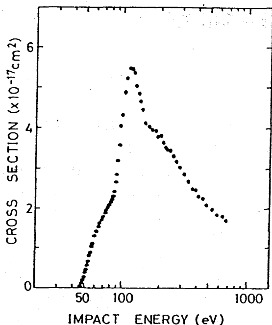
図1. Ba^+ の2重電離断面積
