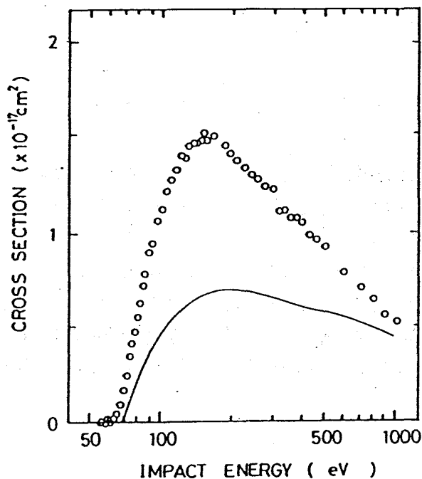
図3. Ca^+ の2重電離断面積. 実線は3S電離+2p電離をLotz の式 (5) で計算したもの
