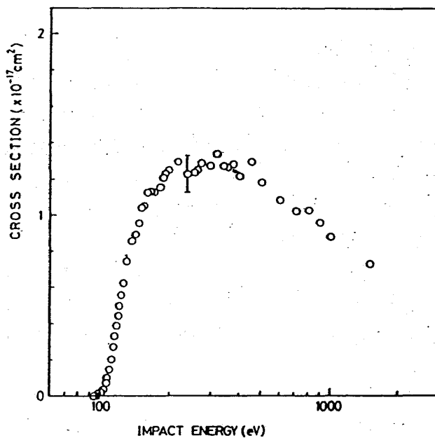
図4. Ba^+ の3重電離断面積
