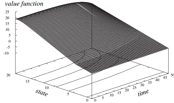
Fig. 1 Value Function
