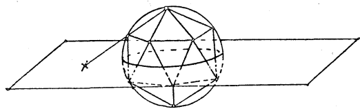
図3. 正20面体の立体射影
