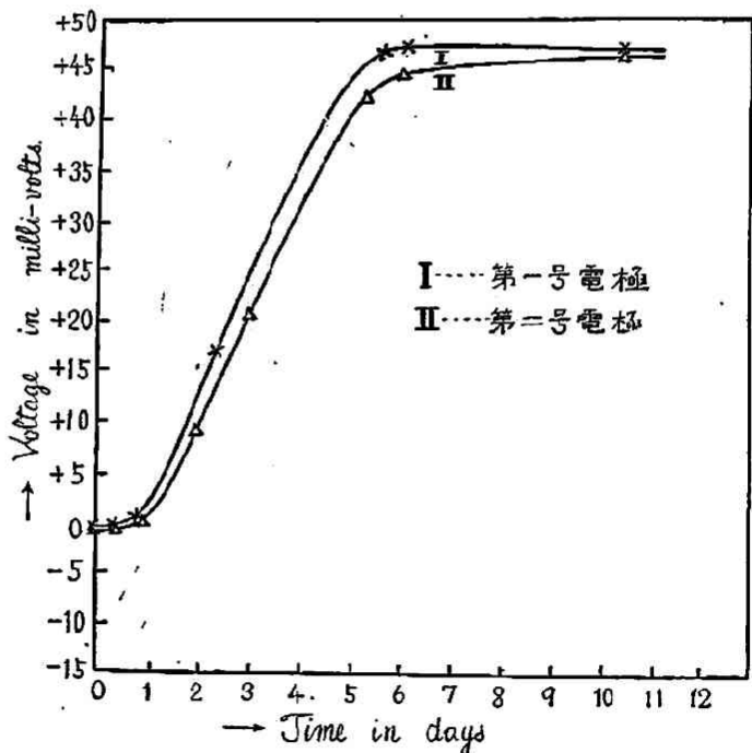
第 六 圖 (酸化銅電極の單極電位の 變化に伴ふ光效果の變化)
