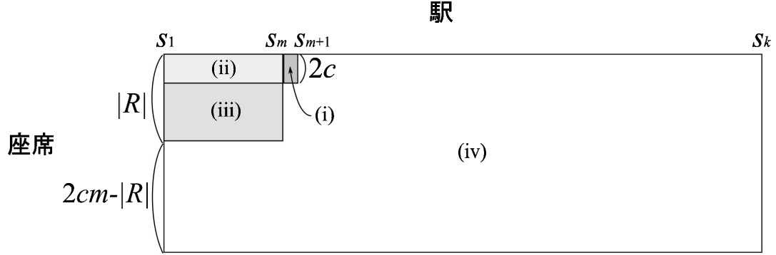
図 3 入力列 \sigma_1 に対するアルゴリズム A の割り当て状況
