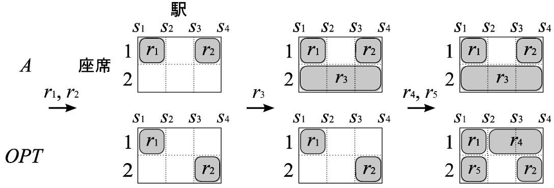
図 2 単一価格問題の例
