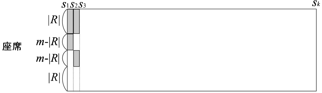
図4 入力列 \sigma_1 と入力列 \sigma_2 に対するアルゴリズム A の割り当て状況
