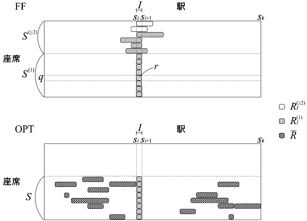
図 5 \sigma に対する FF と OPT の割り当て状況
