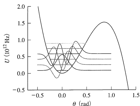
図4 ジョセフソン接合のエネルギー準位量子化. ポテンシャル U , エネルギー準位, 及び対応する波動関数. 計算は \alpha=0.91 , C=75 fF, I_c=60 \mu A の場合.
