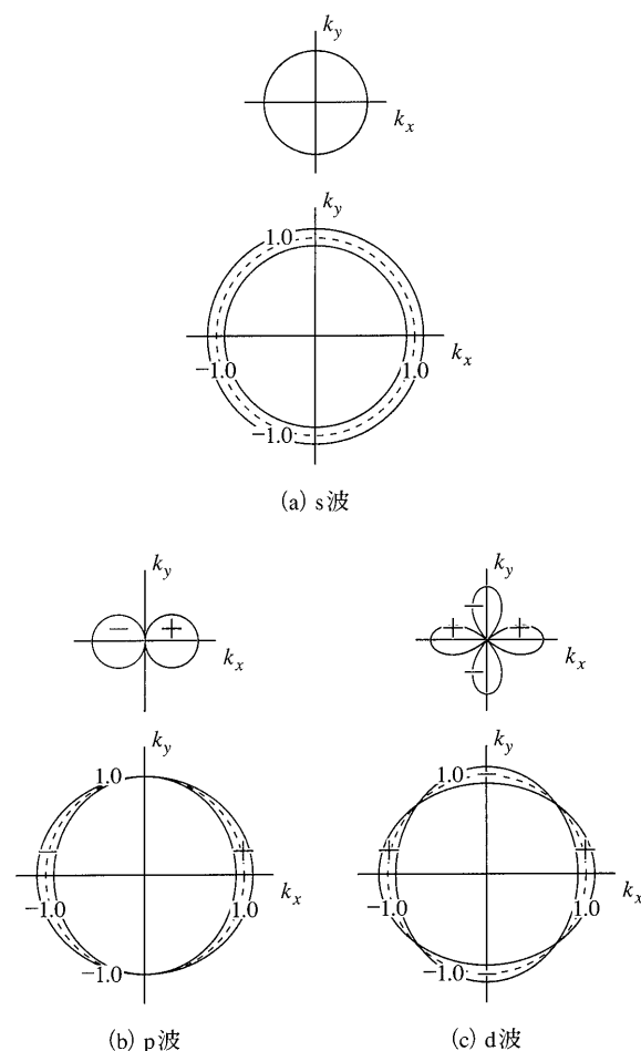
図1 種々の対称性を有する超伝導オーダパラメータ及び超伝導エネルギーギャップの角度依存性
