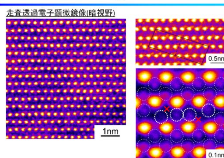
空孔規則相 \text{ReSi}_{1.75} の空孔直接観察
