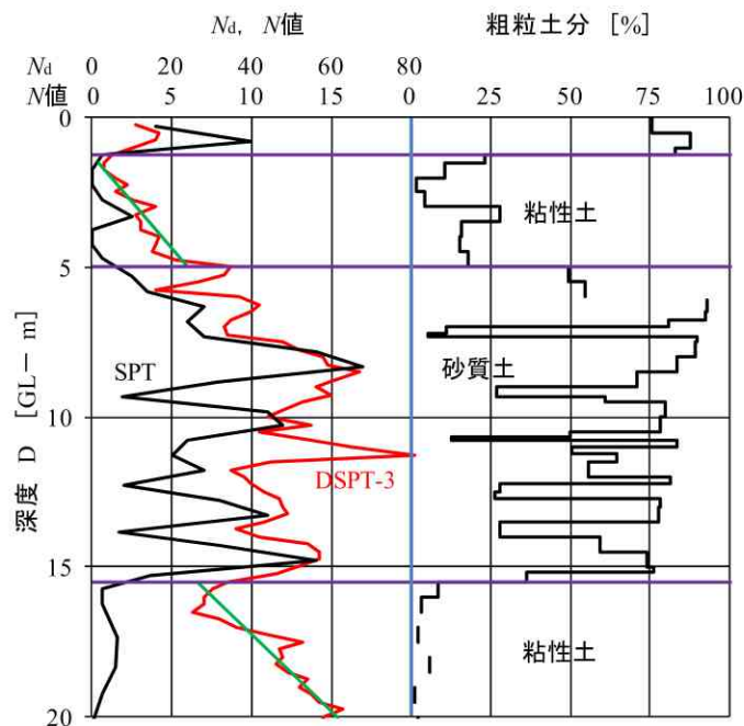
図-3 DSPT-3 の N_d と N 値, 粒度組成の関係
