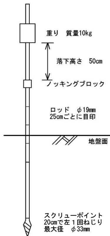
図-1 DSPT試験機の概略図
