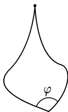
図 2: 端点が一致し, (a, b) 上にカスプが 1 つ存在するフロンタル
