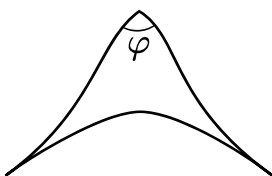
図 3: 端点が一致し, (a, b) 上にカスプが 2 つ存在するフロンタル
