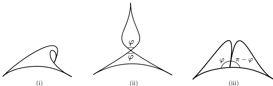
図 4: 自己交差を持つ曲線の図
