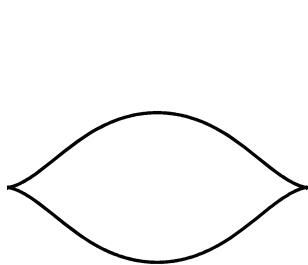
余向き付け可能な波面
