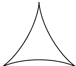
余向き付け不可能な波面
