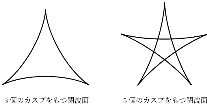
図 5: K(\gamma) = \pi となる曲線
