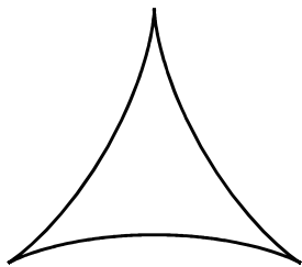
locally L -convex である
