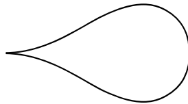
locally L -convex ではない
