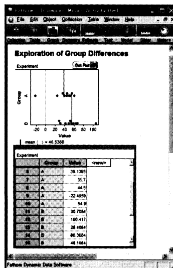
図 18: データ集合
