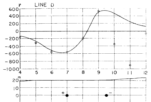
図10 解析結果 (Jorak 地区)
