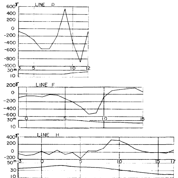
図8 測定結果および地形断面図 (Jorak 地区)
