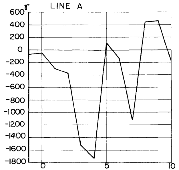
図11 測定結果 (Lenga 地区)
