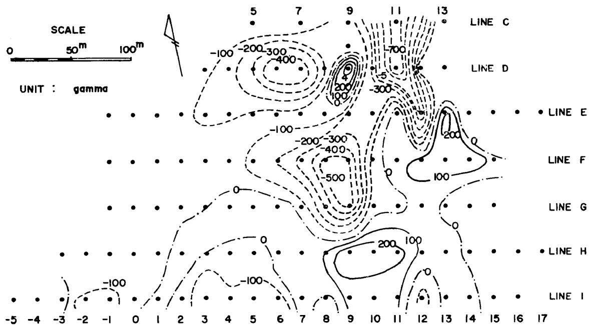
図9 磁力線図 (Jorak 地区)
