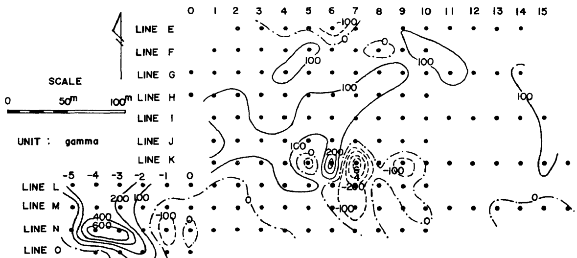
図5 等磁力線図 (Simpang Rengam 地区)
