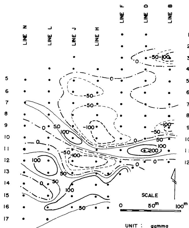
図14 等磁力線図 (Horse Shoe 地区)
