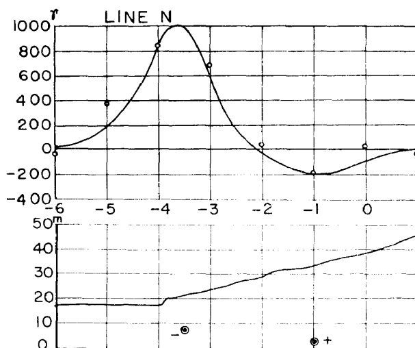
図6 解析結果 (Simpang Rengam 地区)
