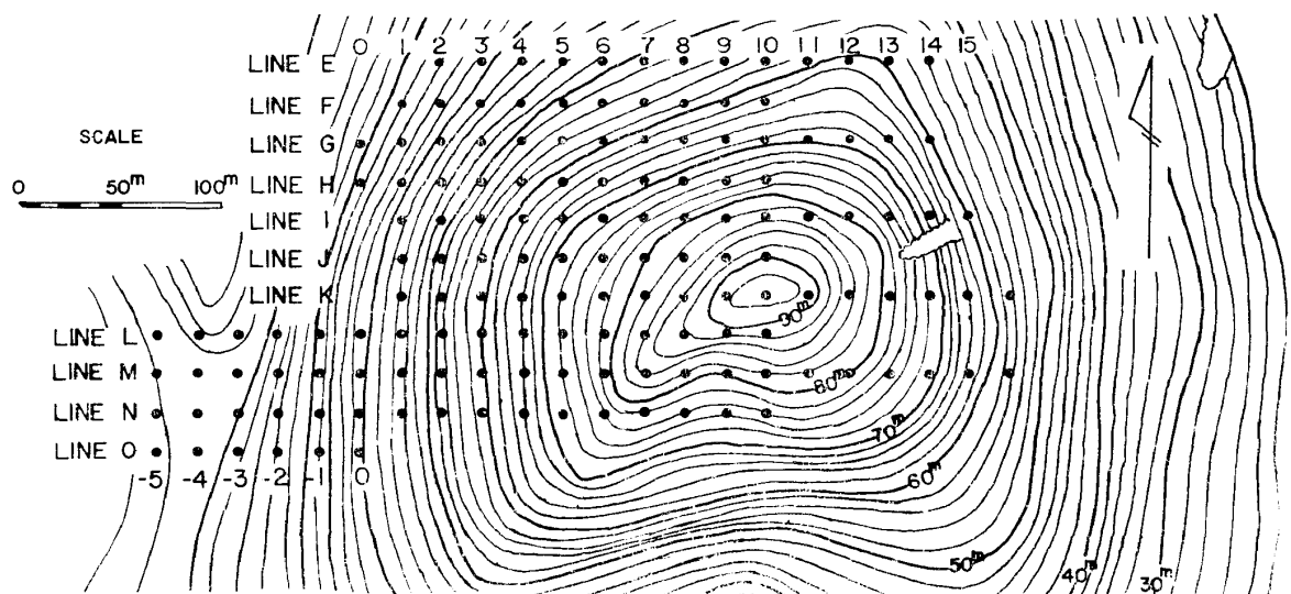
図3 調査地区の平面図 (Simpang Rengam 地区)
