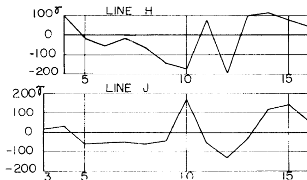
図13 測定結果 (Horse Shoe 地区)
