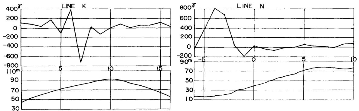
図4 測定結果および地形断面図 (Simpang Rengam 地区)
