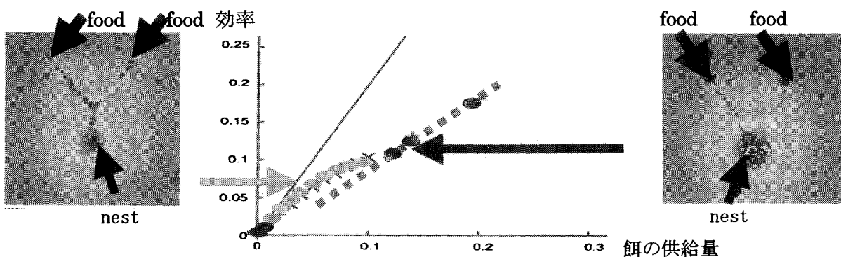
図4. 餌の供給量と効率の関係とそれらに対応する集団の形状
