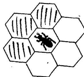
図2. 三角格子上での行動
