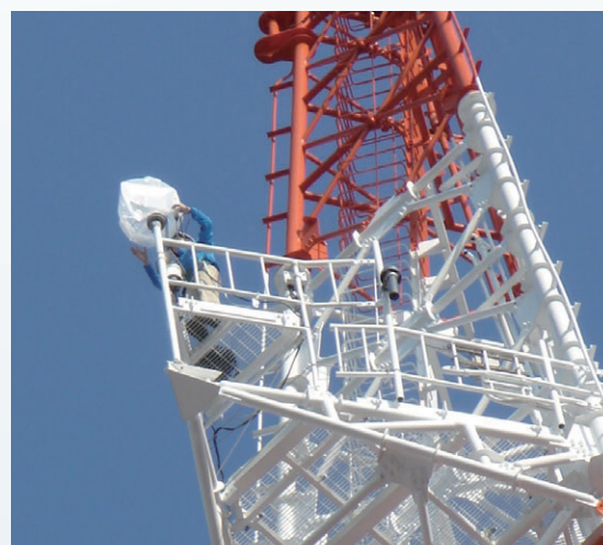
写真2 地上40 mのデッキで超音波風速計に袋をかぶせ、無風状態での値を点検している筆者の様子（技術職員さん撮影）。
