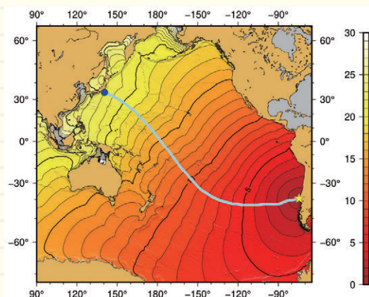
図2 津波先端部の伝播経路推定の一例。色の濃淡は波源から津波が到達するまでの時間(単位:時間)。
