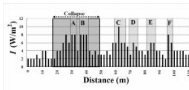
図1 地中音の分布と豪雨後に発生した崩壊の位置
