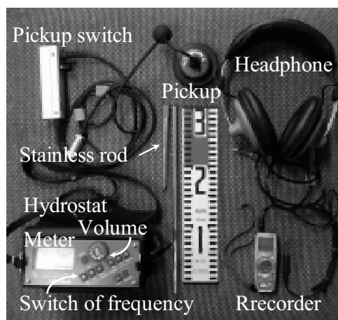
写真1 地中音測定装置
