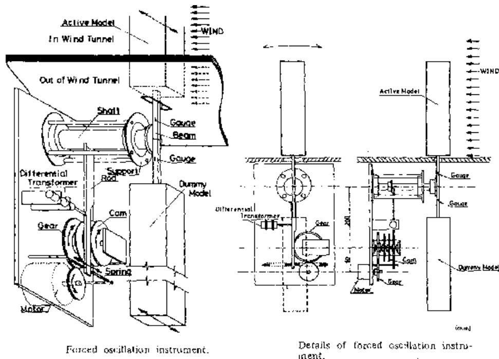
図4 実験装置の概略
