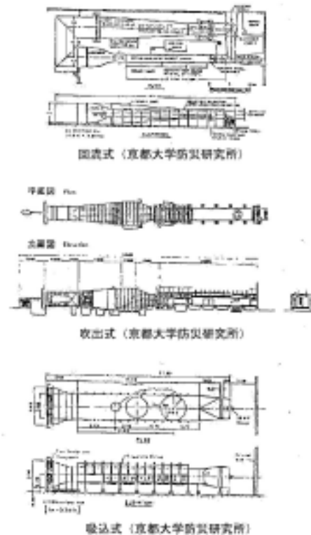
図 1 風洞の種類
