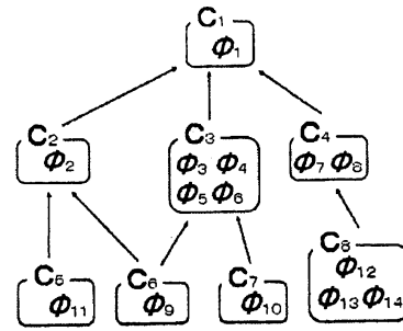
図 5: 階層化されたスキーマベース。ただし、 C_1, \dots, C_8 は次の通り。 C_1 = * \supset * , C_2 = (* \vee *) \supset * , C_3 = * \supset (* \supset *) , C_4 = (* \wedge *) \supset * , C_5 = (* \vee *) \supset \exists * , C_6 = (* \vee *) \supset (* \supset *) , C_7 = (* \supset *) \supset (* \supset *) , C_8 = (* \wedge *) \supset \exists *
