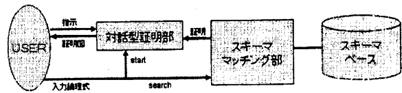
図 6: 本システムの概要
