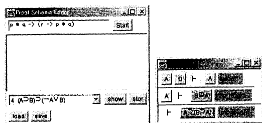
図 7: 論理式の入力(左). スキーマベース内で見つかる有効なスキーマ(右).
