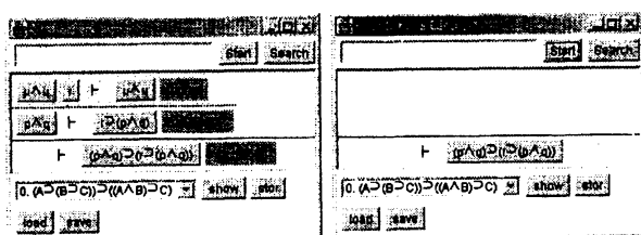
図 8: スキーマを援用して得られた証明(左). スキーマベース内で見つかる有効なスキーマ(右)
