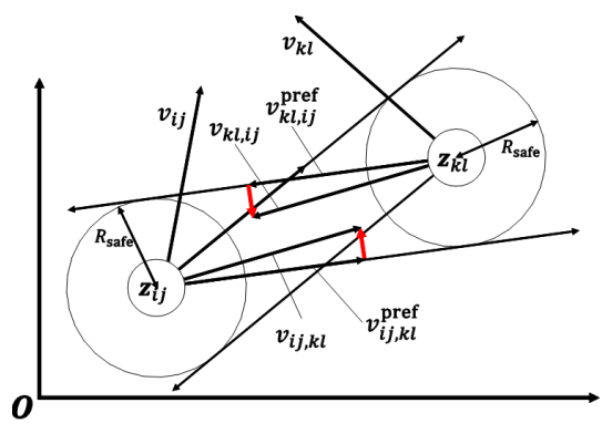
Fig. 4. \mathbf{v}_{ij,kl}^{\text{pref}} and \mathbf{v}_{kl,ij}^{\text{pref}} .
