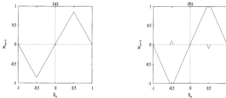
図 4: 対称テントマップの双安定状態(a)( a < 2 ) と単安定状態(b)( a > 2 )。
