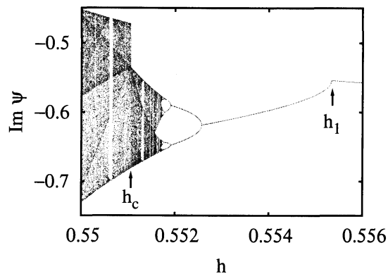
図 1: 分岐図。横軸はコントロールパラメータ h 。縦軸はポアンカレ断面 \text{Re } \psi = 0 かつ \text{Re } \dot{\psi} > 0 での \text{Im } \psi 。
