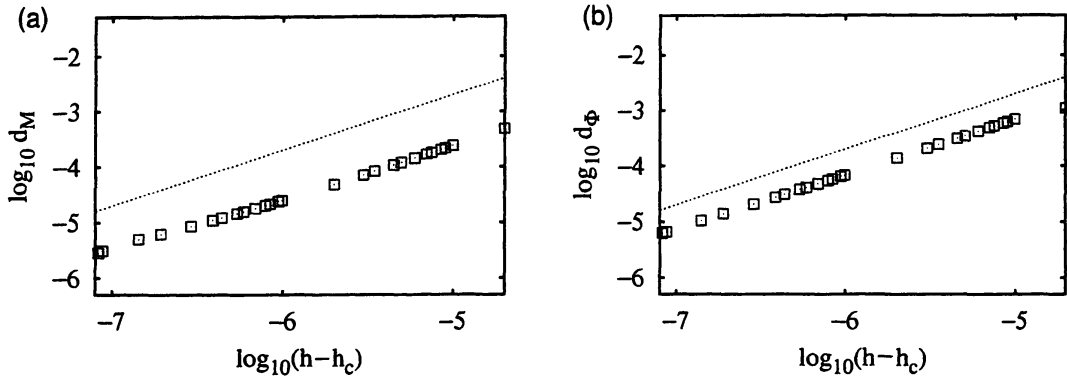
図 3: (a) 距離 d_M の h 依存性。(b) 距離 d_\Phi の h 依存性。いずれも h \rightarrow h_c で線形に減少している。
