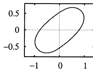
図 2: 媒介解 M を \psi 平面に射影したもの。縦軸は \text{Re } \psi , 横軸は \text{Im } \psi 。
