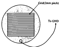
図 4.13: グリッドの概略図
