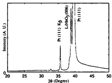
(a) Pt バッファ層 (120nm) 上の LiNbO 3 膜 (LiNbO 3 膜厚: 300nm)
