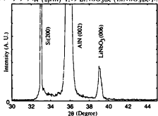
(c) AlN バッファ層 (1.7μm) 上の LiNbO 3 膜 (LiNbO 3 膜厚: 300nm)
