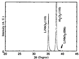
(a) ガス圧: 5mTorr
