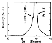
図 3.5: Pt 配向膜上の \text{LiNbO}_3 膜の XRD パターン
