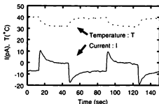
図 4.10: \text{LiNbO}_3 軸配向膜の焦電電流
