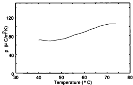
図 3.33: \text{LiNbO}_3 e 軸配向膜の焦電係数
