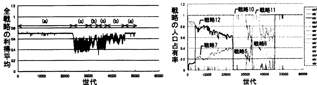
図 3: 2 人信頼度モデル 利得の推移および戦略分布
