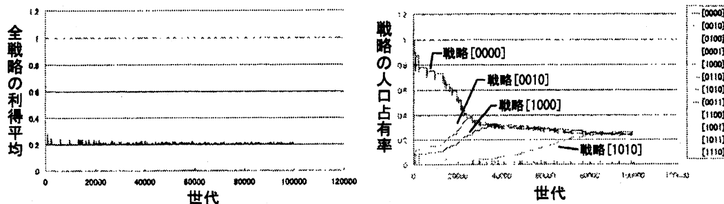
図 4: 5人 Lindgren モデル 利得の推移および戦略分布
