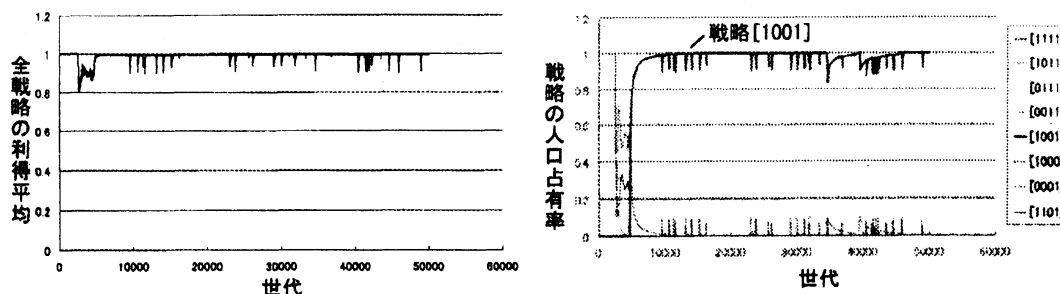
図 2: 2 人 Lindgren モデル 利得の推移および戦略分布
