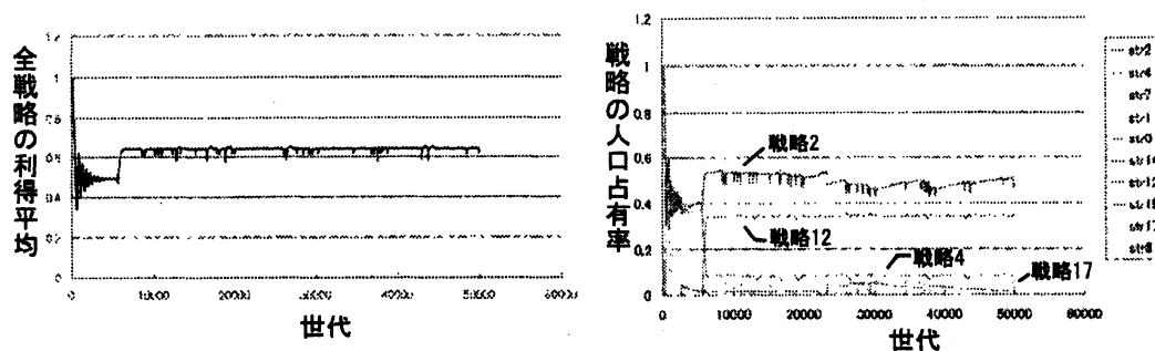
図 5: 5人信頼度モデル 利得の推移および戦略分布
