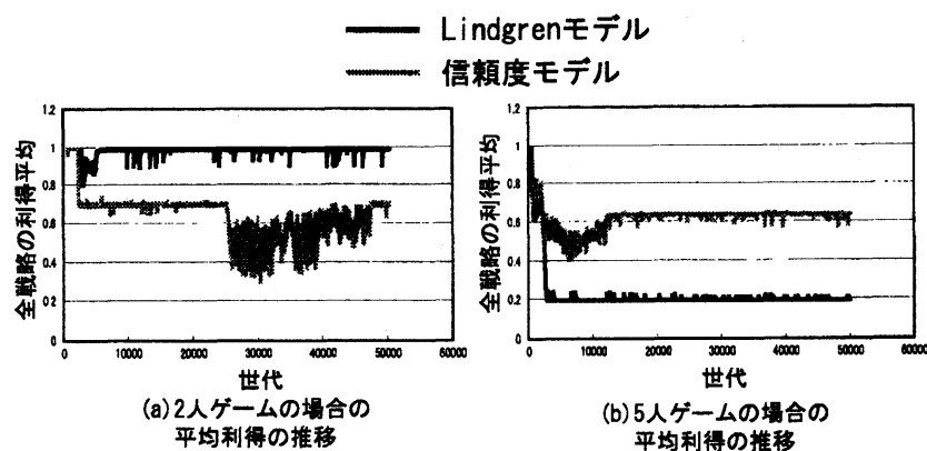
図 6: 2人ゲームと5人ゲームにおける利得の推移
