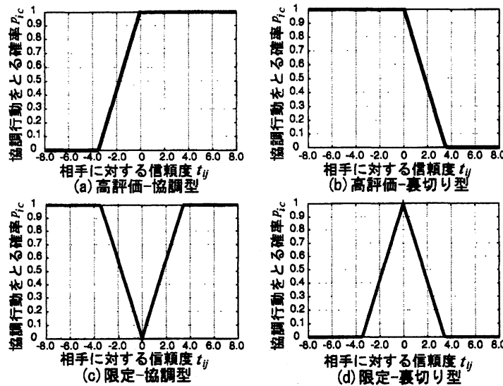
図 1: 行動決定関数一覧
