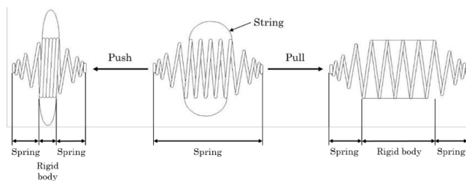
図 15 非線形バネの詳細
