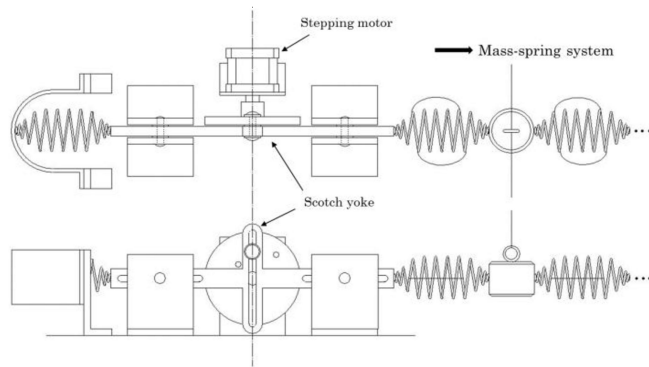
図 17 駆動装置
