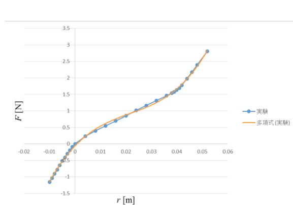
図 3 バネ特性 (実験値と FPU- \beta 系の近似曲線)
