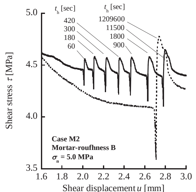
図5 Slide-Hold-Slide型一面せん断試験で得られた岩石不連続面の摩擦抵抗挙動
