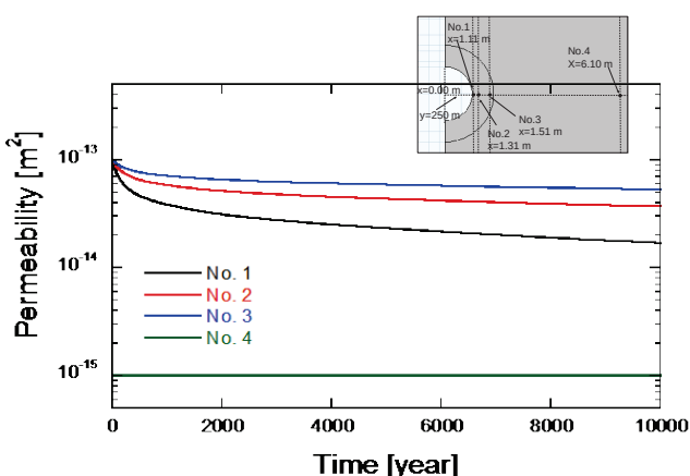
図4 圧力溶解を考慮した空洞周辺の透水性の変化
