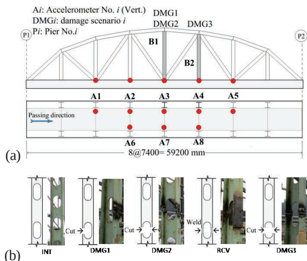
図2 実橋を対象とした損傷検知：(a) 対象橋梁のセンサ配置と損傷部材；(b) 損傷シナリオ
