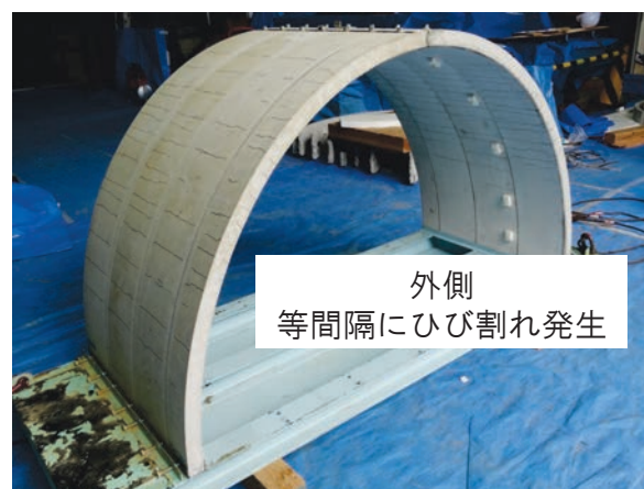
写真1 強震応答振動台実験後のプレキャストアーチカルバート
