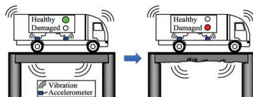
図4 移動橋梁点検の概念
