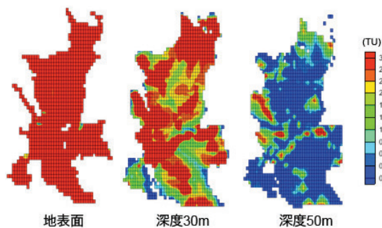
図5 地下水流動解析と物質移行解析による1953年時点での地下水トリチウム濃度の推定分布：京都盆地の例
