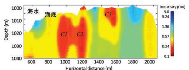
図8 開発した観測機器・インバージョン法による沖縄熱水噴出地域での海底下比抵抗分布：C1～C3の低比抵抗帯は熱水や鉱床の存在を示唆
