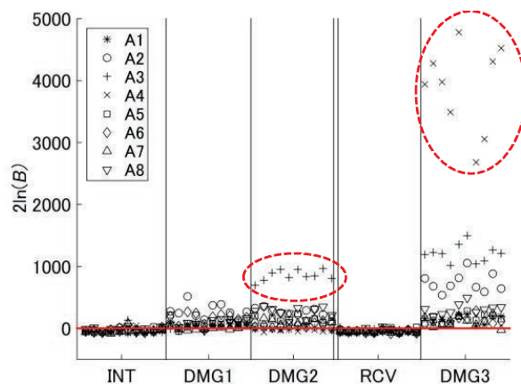
図3 実橋を対象とした損傷検知例
