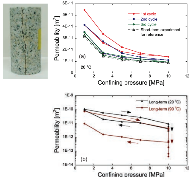
図2 温度・保持時間を変化させた単一き裂を有する花崗岩供試体の透水性と拘束圧の関係
