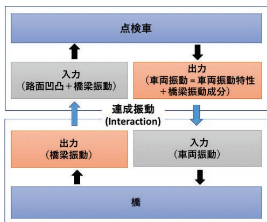
図5 走行車両と橋の動的連成問題の考え方
