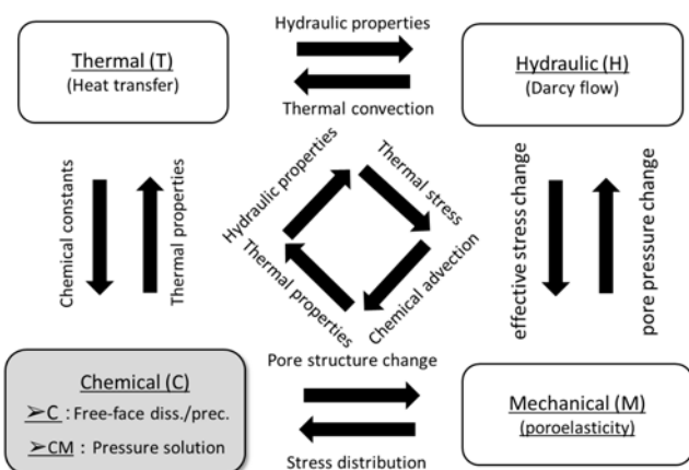
図3 温度(T)-水(H)-応力(M)-化学(C)間の相互作用と連成概念図
