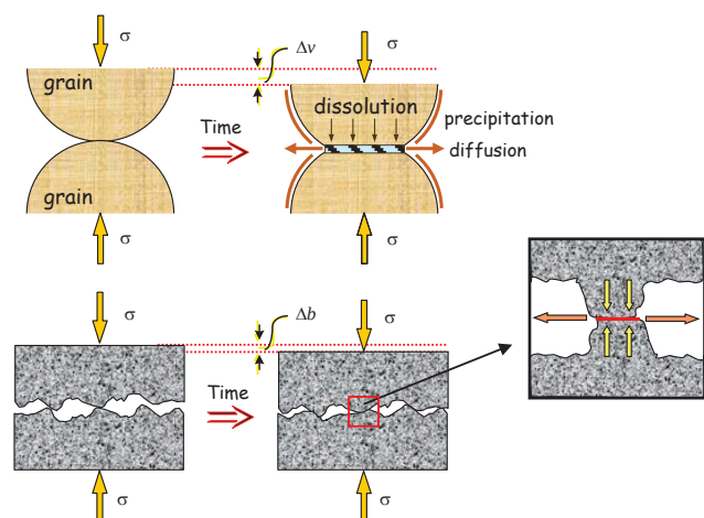
図1 圧力溶解現象の概念図
