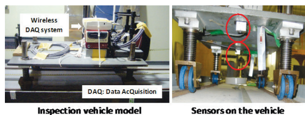
図6 移動橋梁点検のための模型橋梁車両走行実験
