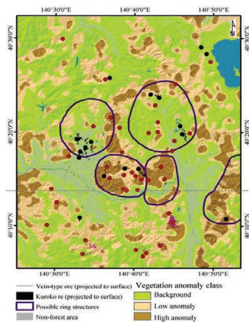
図2 植生指標から示唆される鉱床有望部（茶色）と実際の鉱床の位置：秋田県北鹿・黒鉱鉱床域
