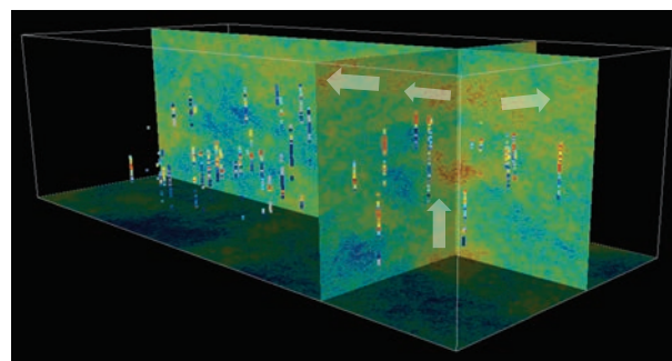
図3 ボーリングデータを用いた地球統計学的シミュレーションによる黒鉱鉱床での銅濃度分布（寒色が低濃度で暖色が高濃度）と鉱液の推定パス（矢印）
