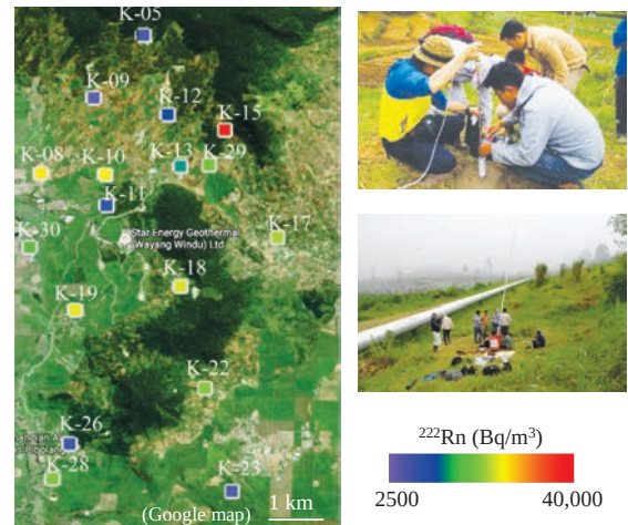
図6 Wayang Windu 地熱地区でのラドン濃度分布（左）、および計測井の設置と測定の様子（右）
