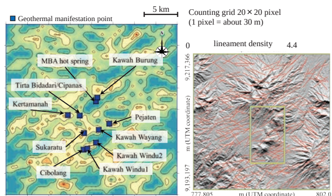
図1 亀裂情報の高精度抽出例：Wayang Windu 地熱地区（インドネシア）でのリニアメント密度マップと地熱兆候点の分布
