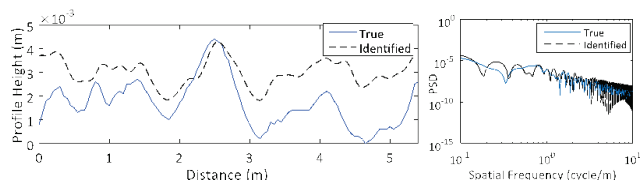
図7 模型実験の車両振動による路面凹凸同定例
