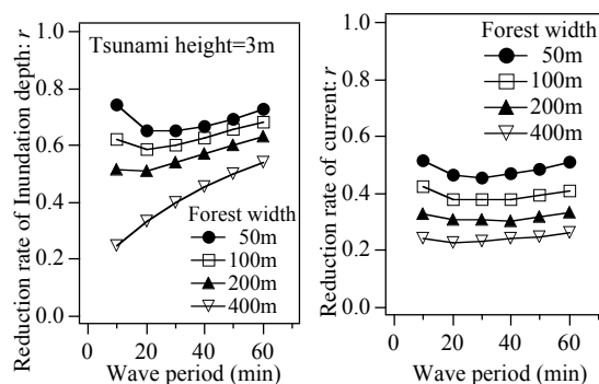
Fig. 2 津波周期と津波低減効果
