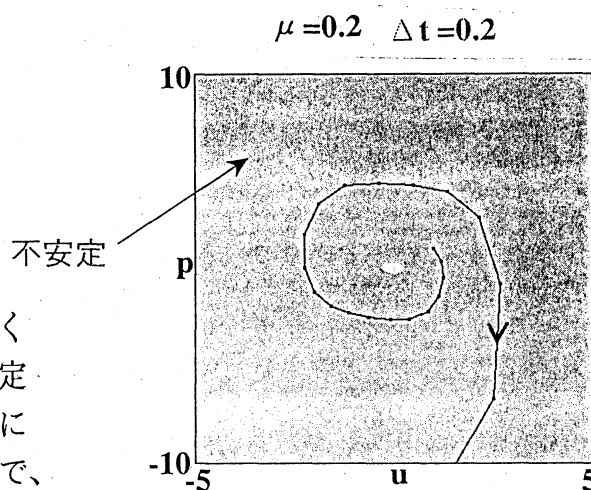
図4 オイラー法
