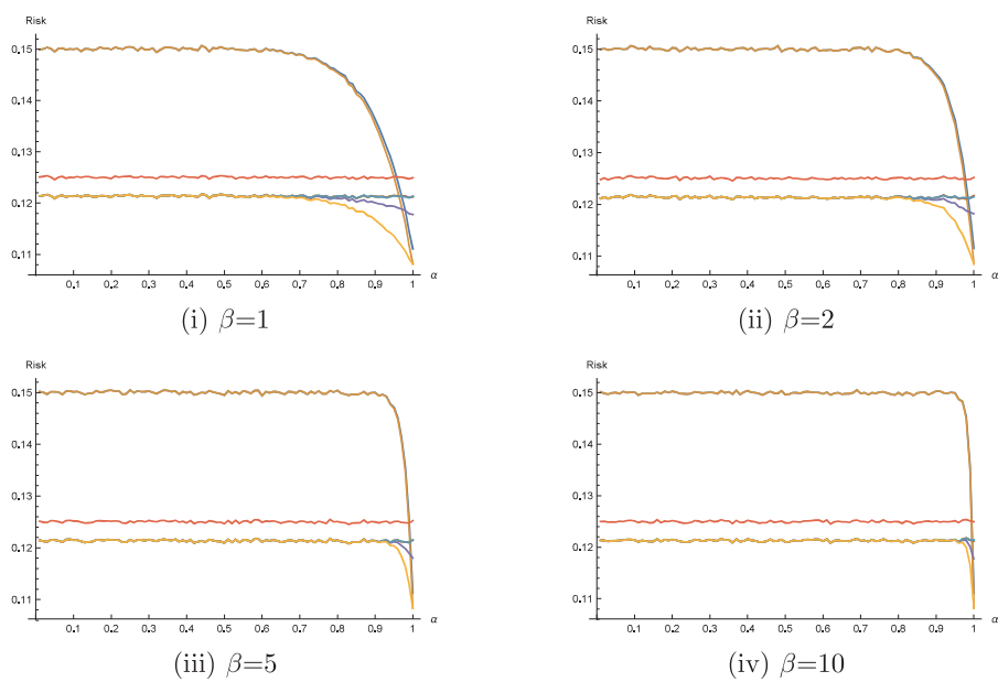
図 9. シンメトリック損失関数 ( n = 10 )
