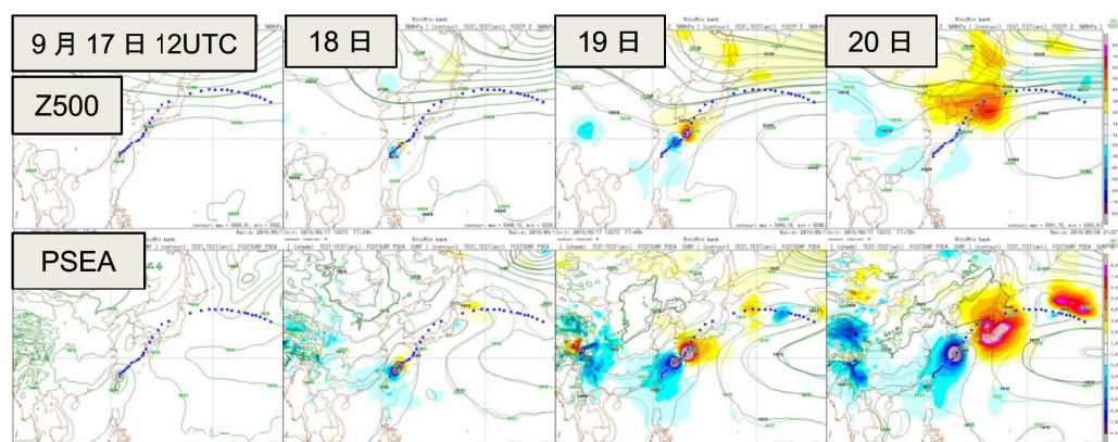
図 6 2016 年 9 月 17 日 12UTC から 20 日 12UTC における 500hPa 高度[m](上)、海面更正気圧[hPa](下)と台風第 16 号の予測進路(共通)。黒線は 17 日 12UTC 初期値での予測値、緑線は解析値、カラーは予測値からの解析値の差分(赤色が正)、ドットは予測進路を表す。
