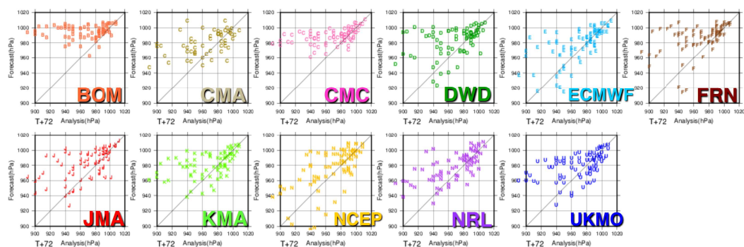
図 4 縦軸に 72 時間予報の中心気圧[hPa]、横軸にベストトラックの中心気圧[hPa]を描いた散佈図。各数値予報センターについて北西太平洋域のものを示す。
