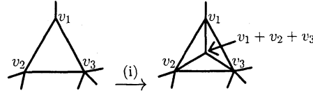
図 2: 操作 (i).
