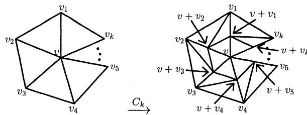
図 4: 操作 C_k .
