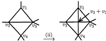
図 3: 操作 (ii).
