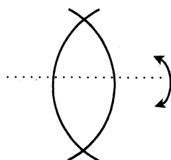
図 8.7 C_2 の作用
