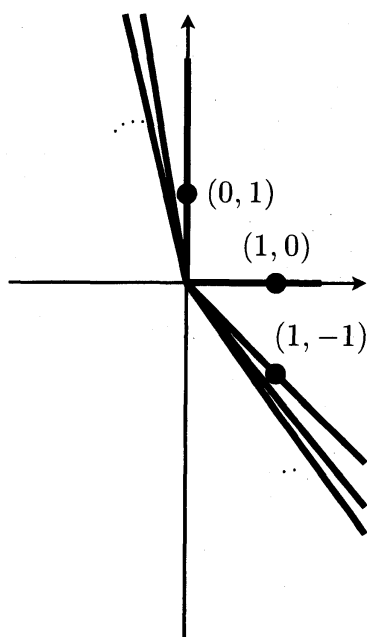
図 8.4 扇 \Sigma
